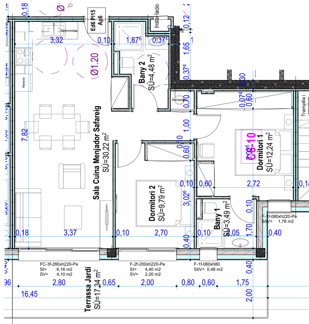
Ed6 PI15 Ap5 (s/Terr.) Ed6 PI15 Ap5 (a/Terr.) SC=69,84 m 2 SC=87,46 m 2
